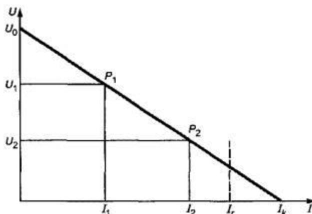
P_1, P_2 - точки, построенные при измерении нагрузочных характеристик
