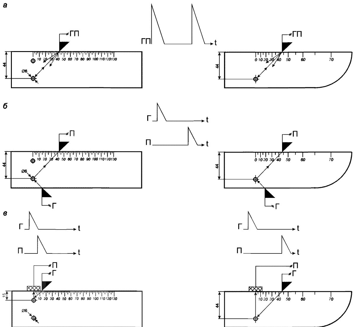
Рисунок 5 — Схема расположения преобразователей на стандартном образце СО-2Р (СО-3Р) при измерении (настройке) условной чувствительности при контроле: а — эхо-методом, б — зеркальным методом, в — дельта-методом
